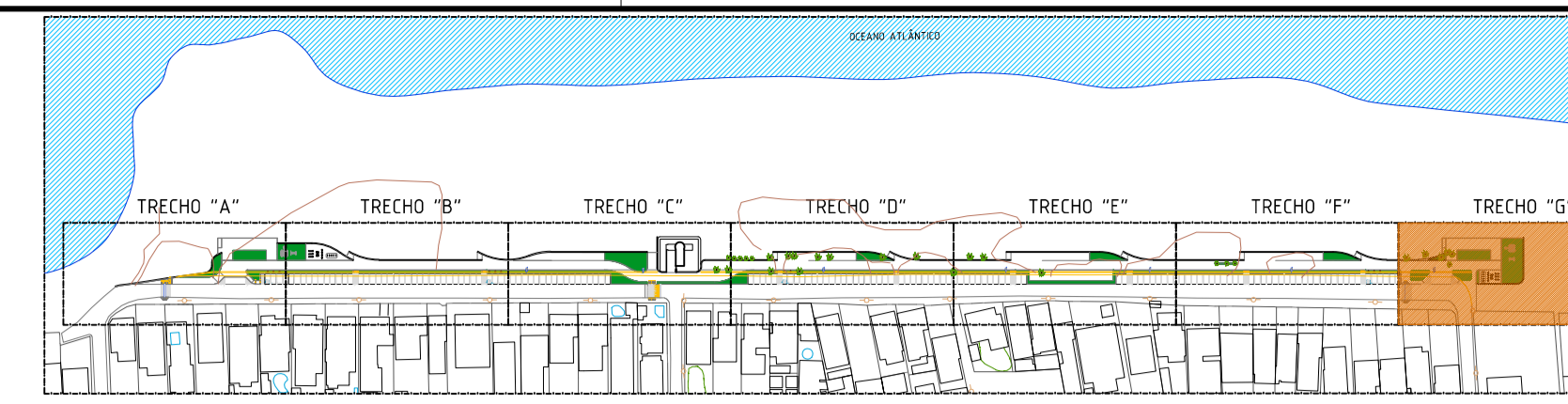
PLANTA COM DEMONSTRATIVO DAS AMPLIAÇÕES ESCALA: 1/3.000
