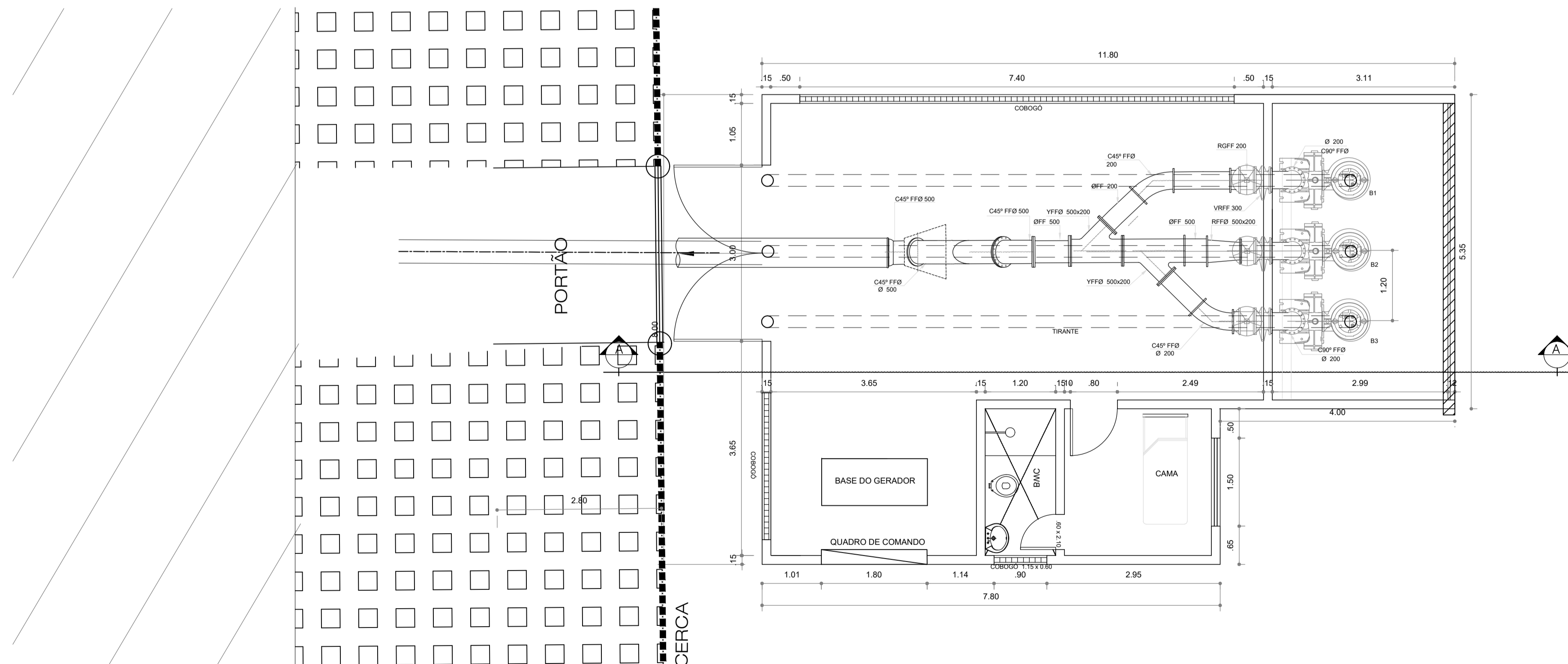
PLANTA BAIXA DA ESTAÇÃO ELEVATORIA DO RD4 ESCALA 1:50
